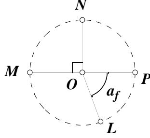
Fig. 11. D''_{f+1}(F) .
