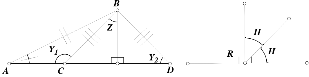
Fig. 6. D_0(F)
